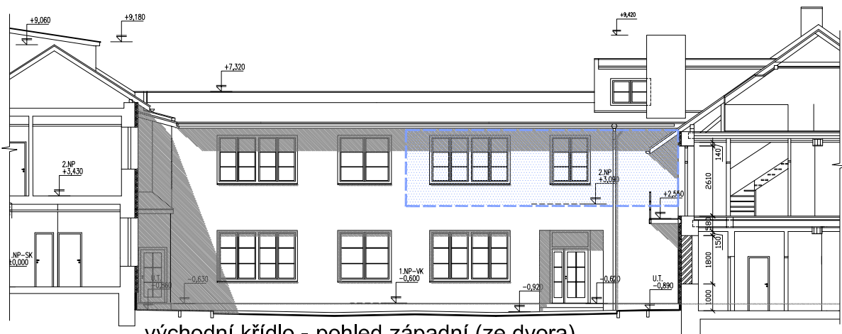
východní křídlo - pohled západní (ze dvora) s vyznačením plochy bytu, M 1:200
