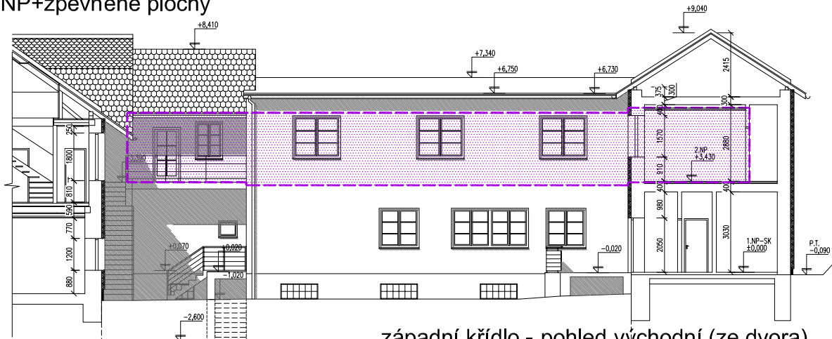
západní křídlo - pohled východní (ze dvora) s vyznačením plochy bytu, M 1:200
