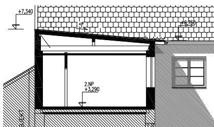
řez M 1:200
